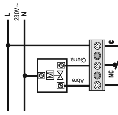
Conexión con una válvula motorizada
