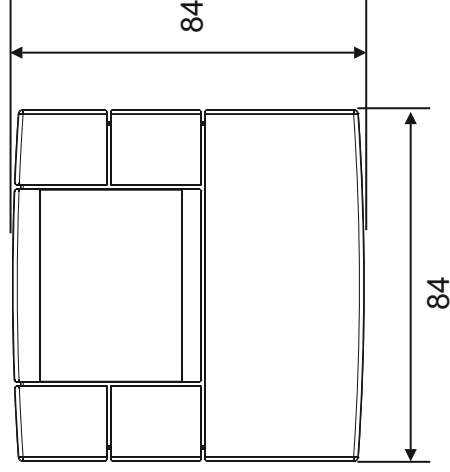
Installation murale sur boîtier à encastrement rond
