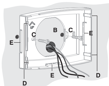
Base per installazione a parete del termostato
